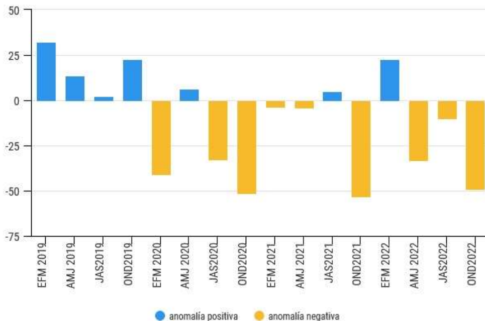
Figura 4. Anomalías trimestrales a escala país desde 2019 al 2022
