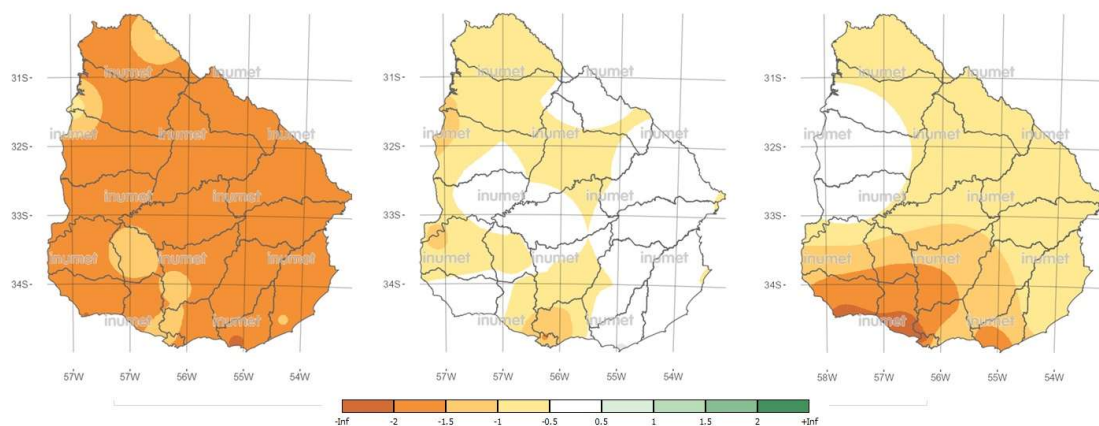
Figura 3. Índice estandarizado de precipitación de 12 meses, 2020 al 2022 de izquierda a derecha.
