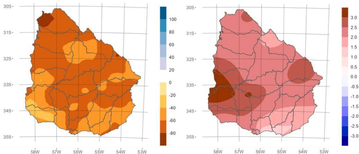
Figura 5. Anomalías en Noviembre Diciembre 2022 y Enero 2023 de precipitación (izq.) y temperatura máxima (der.).
